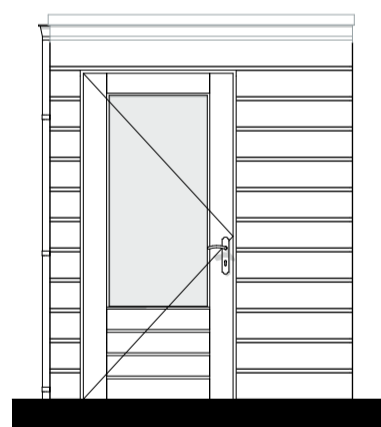
Achtergevel
