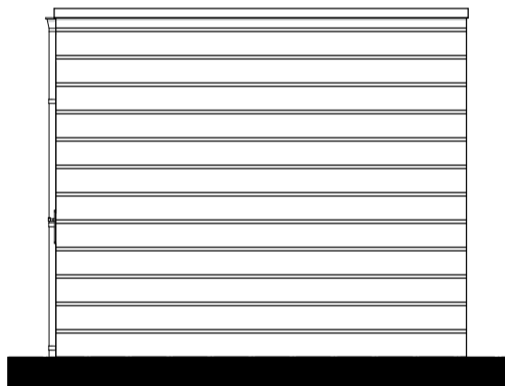
Achtergevel 1:50
