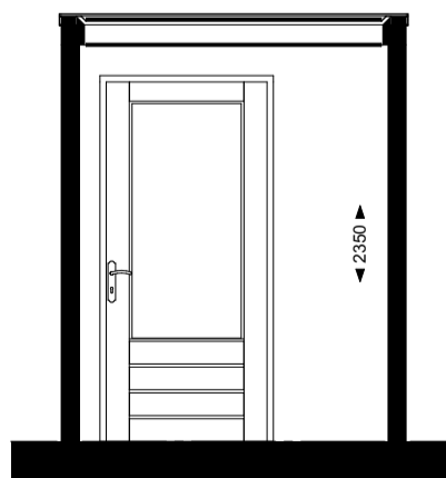
Doorsnede B-B 1:50
